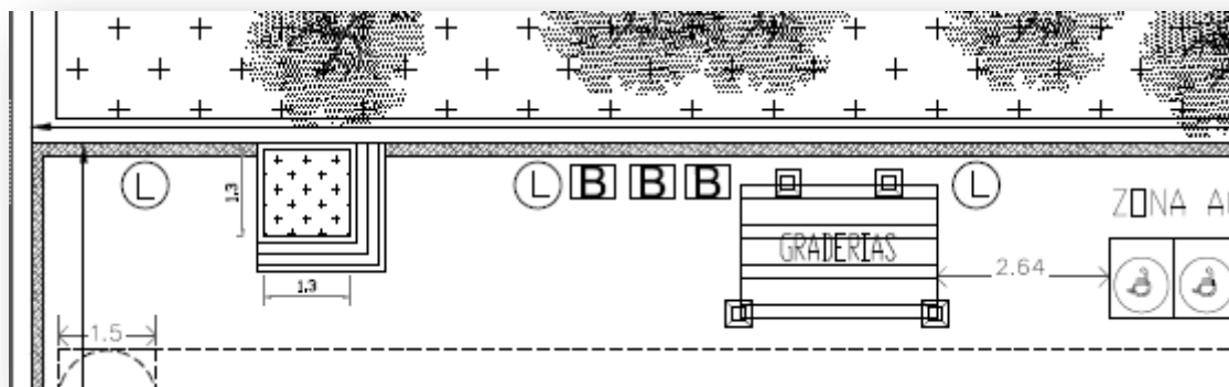
Tramo A B planimetría Original, simbología Luminaria (L)
